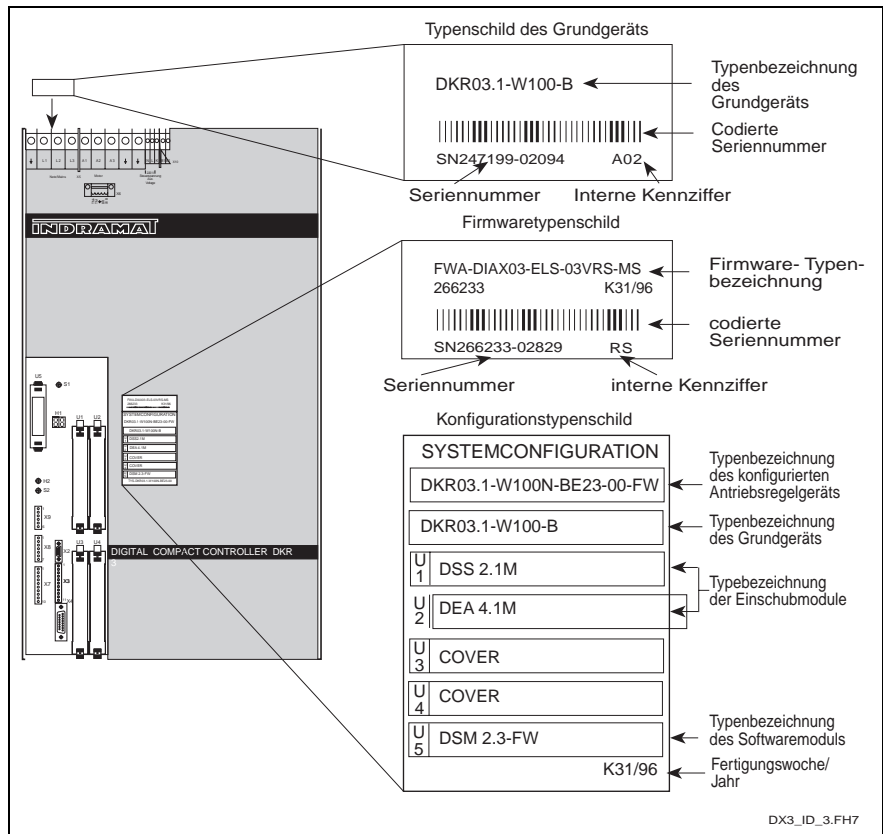
Abb. 4-3: Typenschilder des DKR03.1 (Beispiel)
