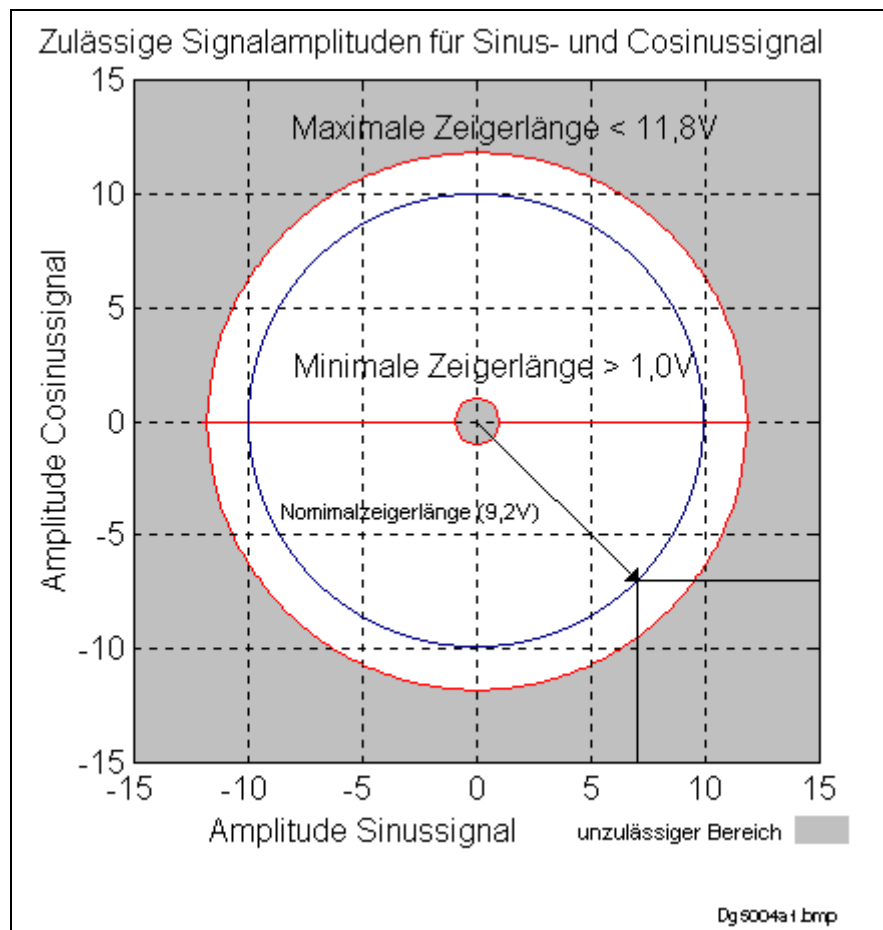
Abb. 2-6: ordnungsgemäße Signalamplitude
