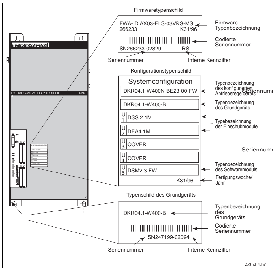
Abb. 4-4: Typenschilder des DKR02.1 bzw. DKR04.1 (Beispiel)
