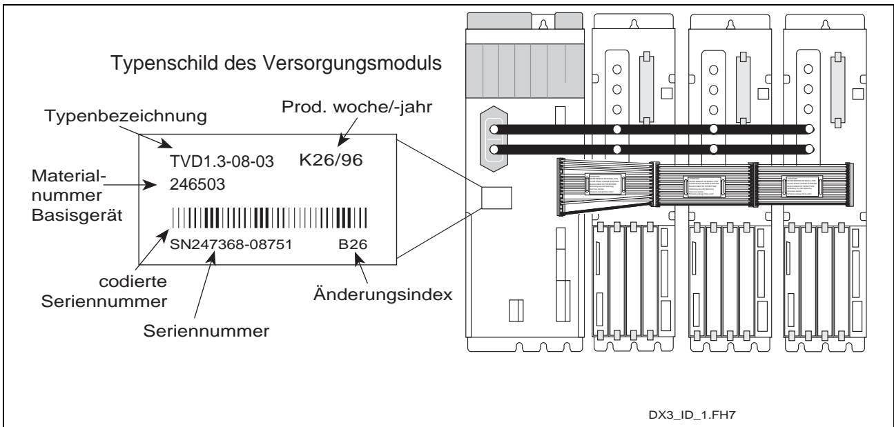
Abb. 4-1: Typenschild am Versorgungsmodul (Beispiel)
